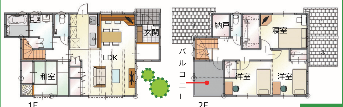
平面図
